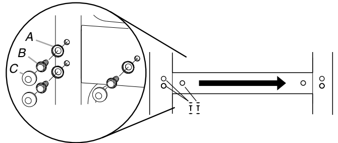
A. Rondelle des chapeaux bombés B. Vis de charnière à tête hexagonale \frac{5}{16} " C. Chapeaux bombés
