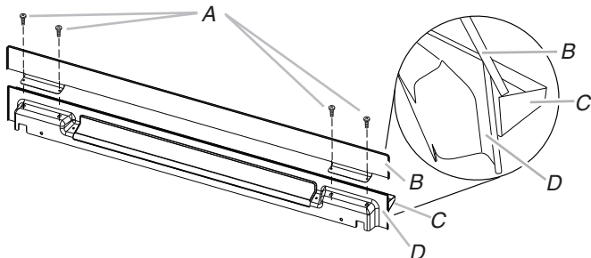
A. Vis n° 8-18 x \frac{1}{4} " B. Garniture de l'évent inférieur C. Pièce d'évent supérieure D. Pièce d'évent inférieure
