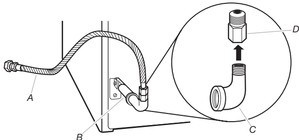
A. Conector flexible de gas de 3/8"
